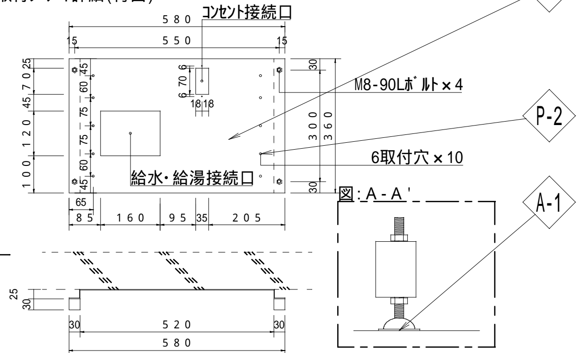
取付プレート詳細(背面)
