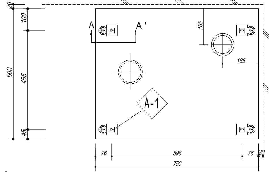
アンカー及び排水位置図
